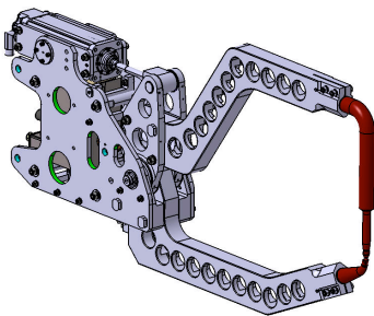
17 Schweißzangen mit Alu Zangenarme
